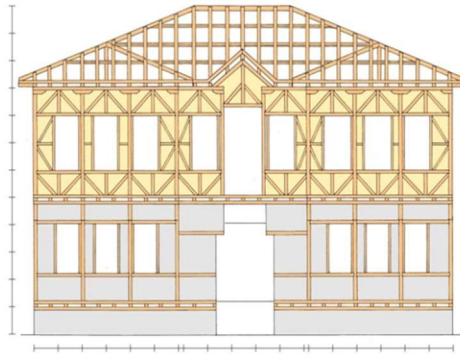
Το κατασκευαστικό σύστημα του αρχοντικού Χάρη. Διακρίνονται οι ξυλόπηκτες τοιχοποιίες στον όροφο, όπου φαίνεται ο ξύλινος σκελετός 3
