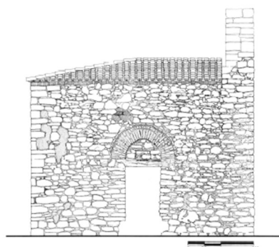
Νοτιοανατολική όψη του κουλέ 4
