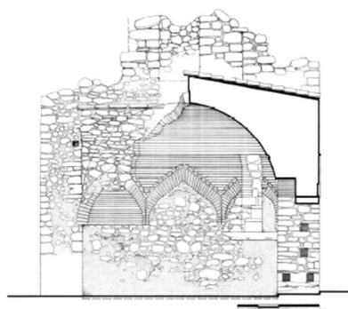
Κατά μήκος τομή του κουλέ 5
